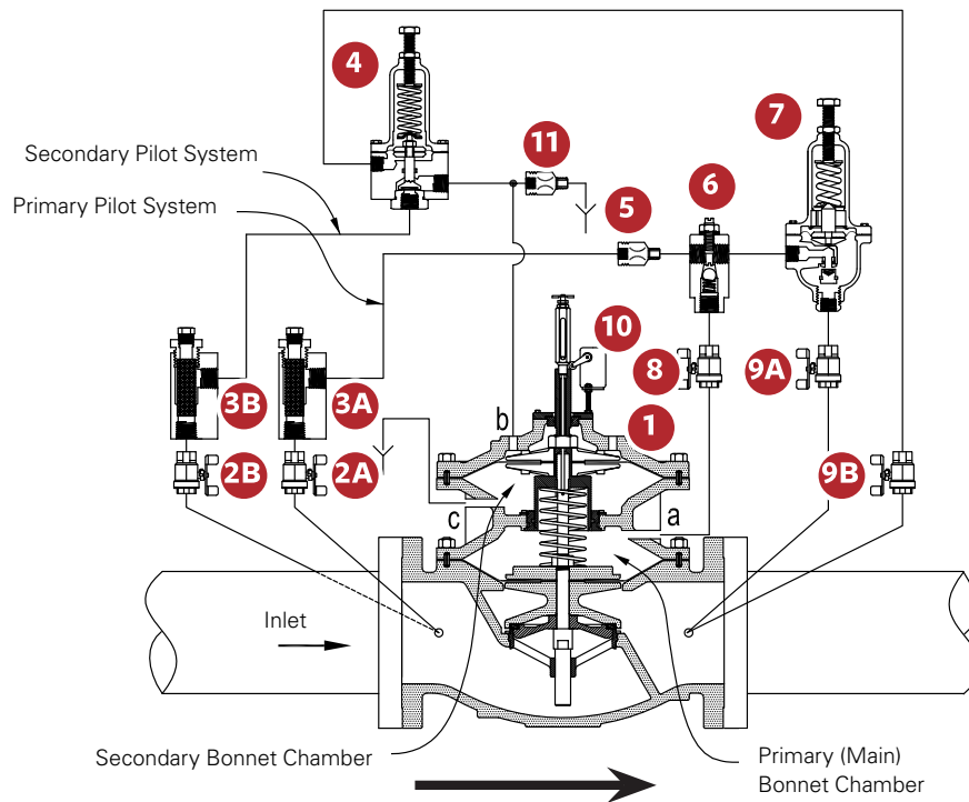
FIG. 2 Schematic A-7697D
