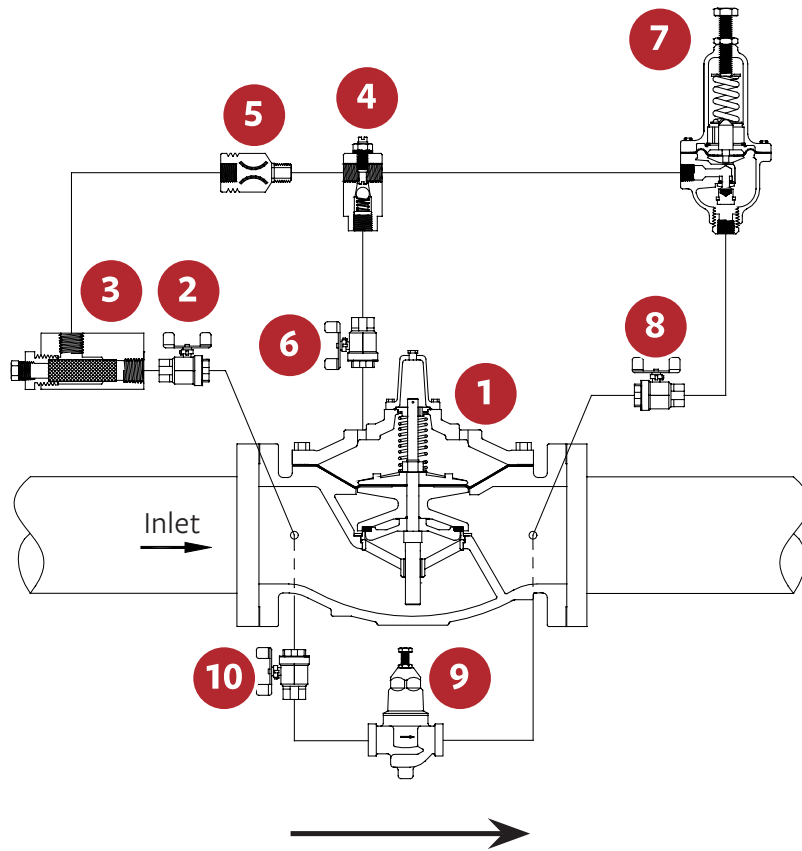
FIG. 2 Schematic A-8063E
