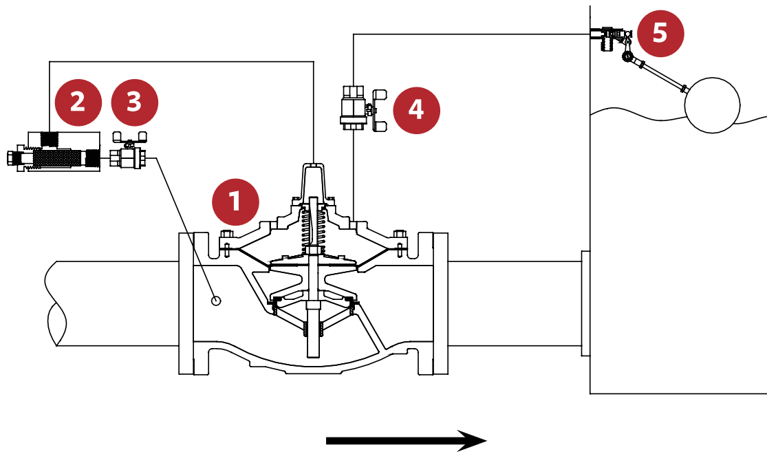
FIG. 2 Schematic A-0593C
