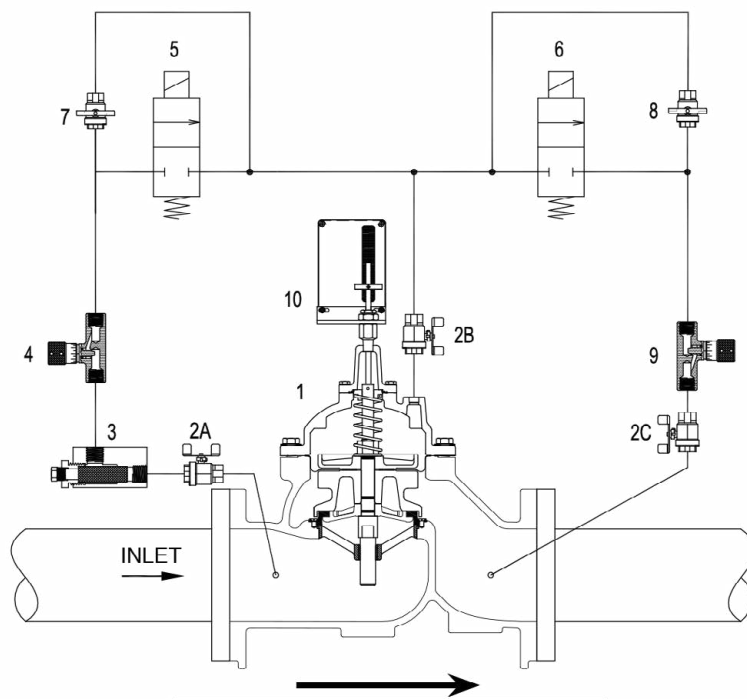
FIG. 2 Schematic A-7637A
