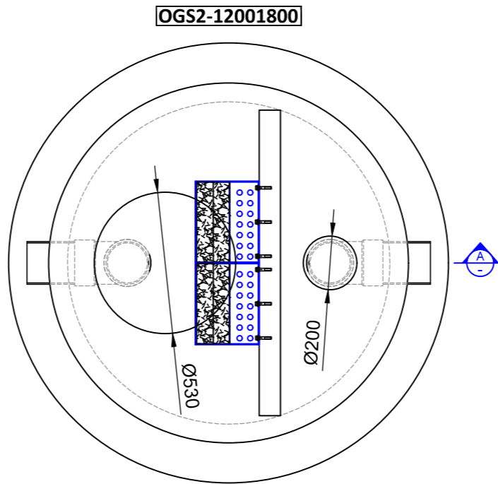
Plan Scale: 1:20
